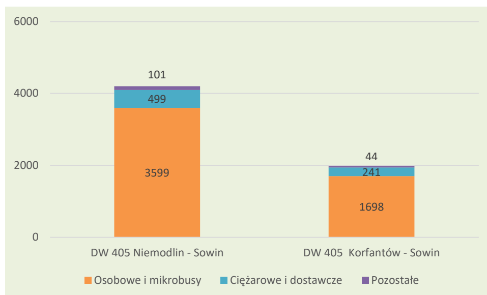
Wykres 20: Średnia dobowa liczba pojazdów na odcinkach drogi wojewódzkiej nr 405 w odniesieniu do gminy Tułowice (2015)
